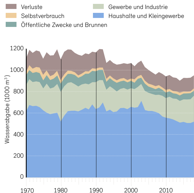
Abb. 7-1: Entwicklung der Wasserabgabe in der Schweiz 1970 – 2018 Dargestellt ist die Wasserabgabe nach Verwendung über die Zeit. Der Verbrauch ist seit den 1990er-Jahren leicht rückläufig, steigt aber in den letzten Jahren wieder an.
