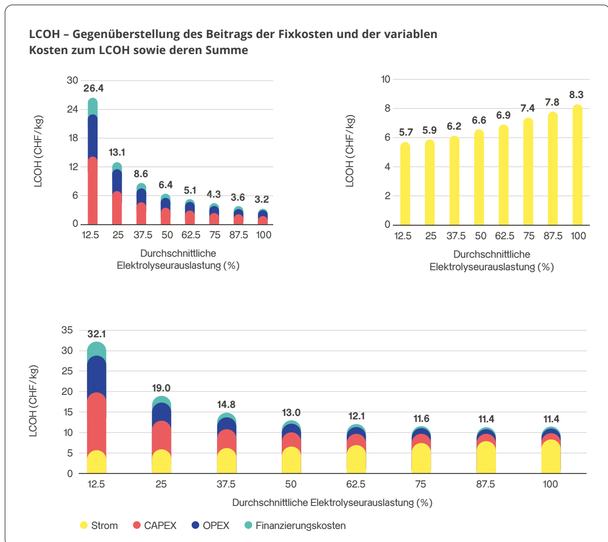
Abbildung 4: Beitrag der Fixkosten (links oben) und der variablen Kosten (rechts oben) zum LCOH sowie die Summe beider Kostenkategorien (unten), in Abhängigkeit der Elektrolyseauslastung
