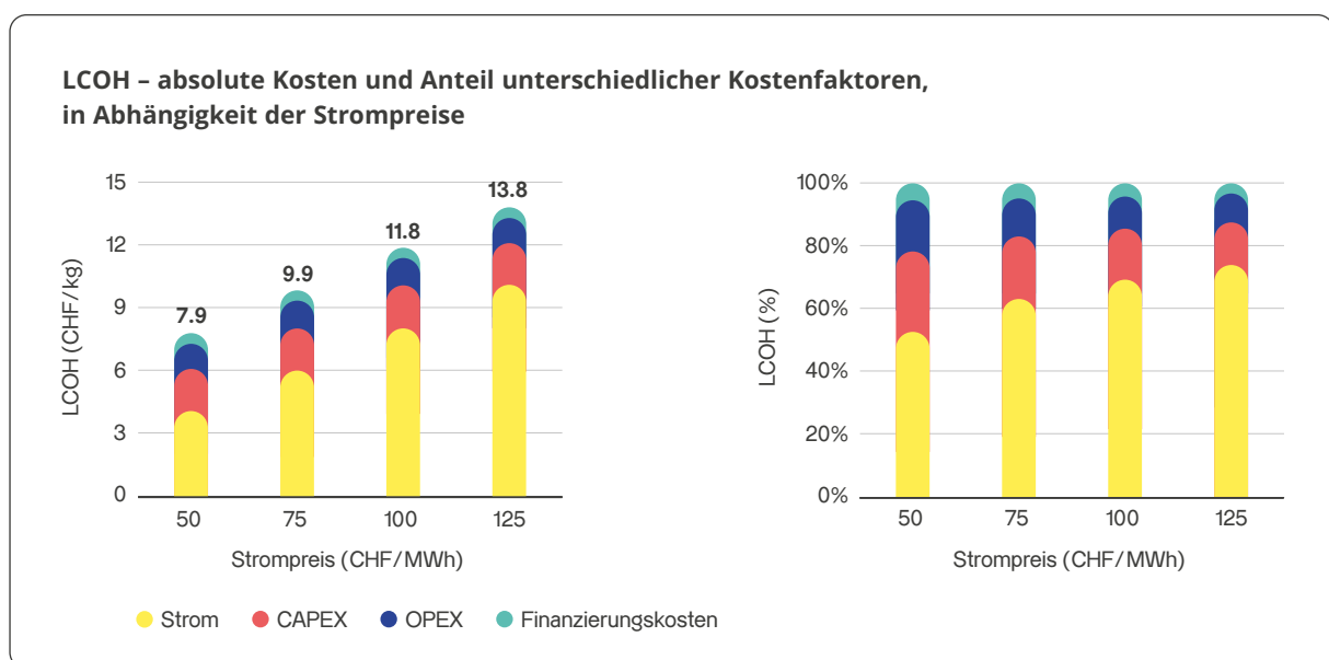
Abbildung 3: LCOH in Abhängigkeit des Strompreises (links); prozentuelle Anteile unterschiedlicher LCOH-Kostenfaktoren bei unterschiedlichen Strompreisen (rechts)
